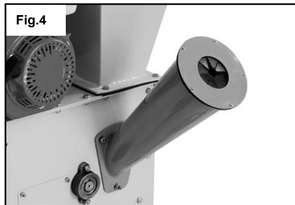
Fig.4 Installation de l'entonnoir
